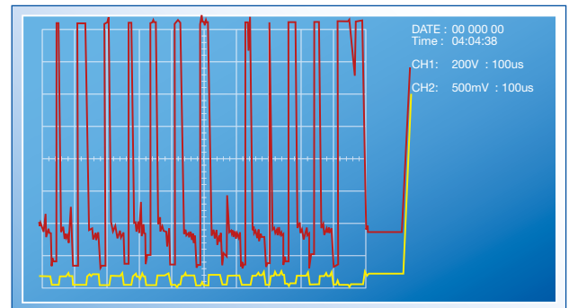
Encendido regular para el mecanizado fino con IonoPlus IME-MH
