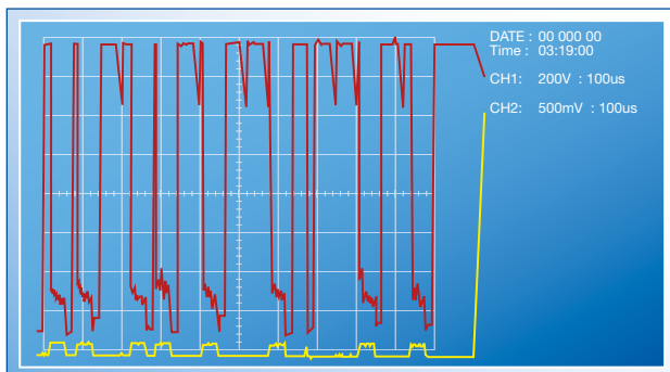
Encendido irregular durante el mecanizado fino
