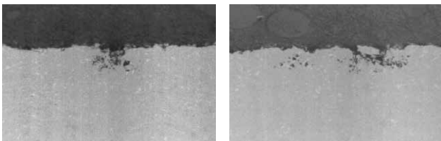
La imagen superior muestra claramente las áreas donde el agua ha dañado significativamente la superficie debido a la lixiviación del cobalto.
