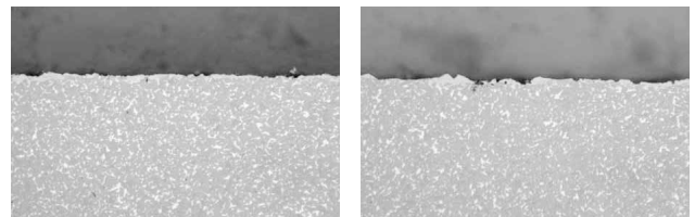
Superficie intacta, mecanizada con IonoFil
